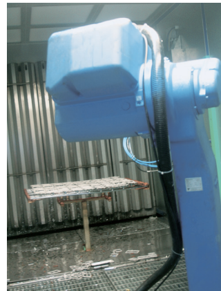
7 - Particolare della cabina di verniciatura robotizzata
